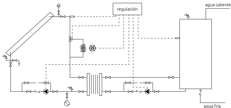
Figura 17. Esquema con energía solar térmica IMS (CPC solar).
