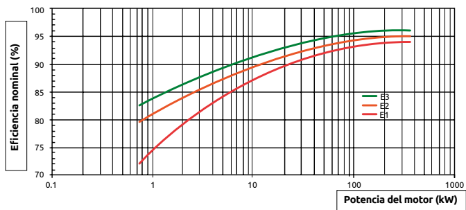
Figura 14. Comparación de las curvas de eficiencia energética de los diferentes tipos de motores (CIRCE, 2013).
