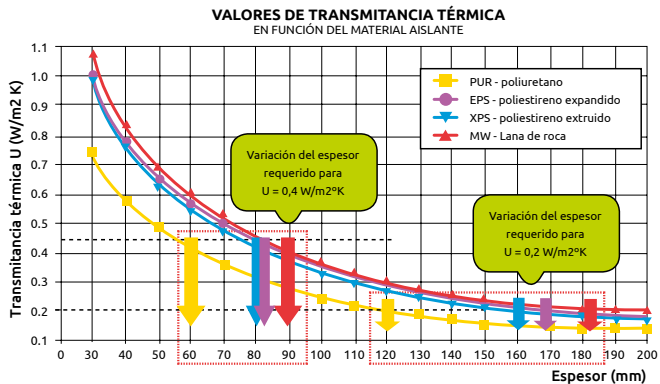
Figura 13. Transmitancia térmica de diferentes materiales y espesores.
