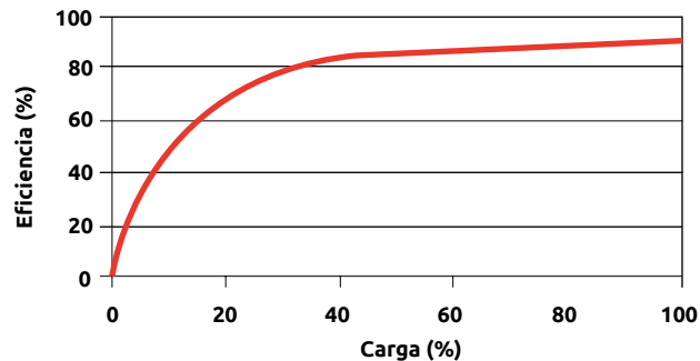
Figura 15. Eficiencia de un motor eléctrico en función del nivel de carga (BREF, 2009).
