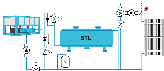
Figura 11. Esquema de un proceso de almacenamiento de frío en paralelo con el sistema de enfriamiento (CIAT).
